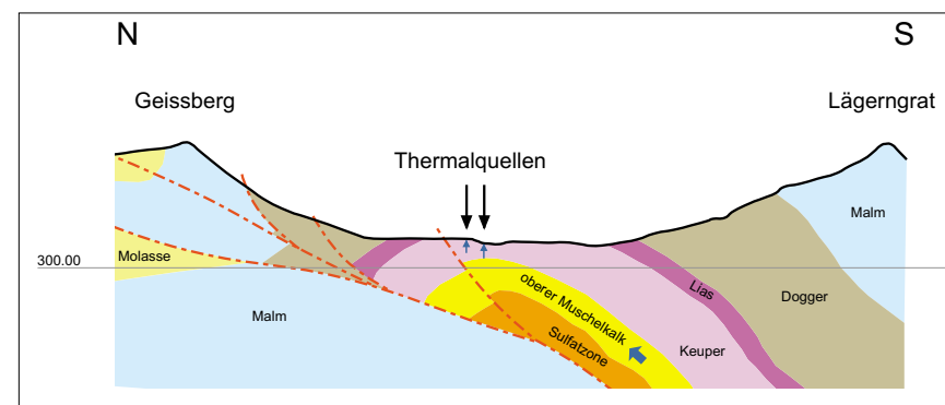
Querprofil durch die Badener Klus
